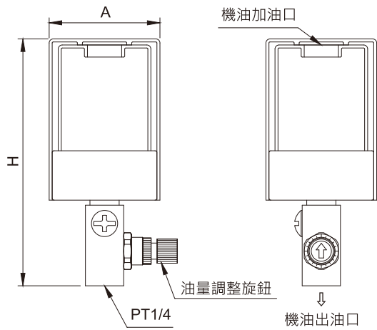
OP 外型圖
