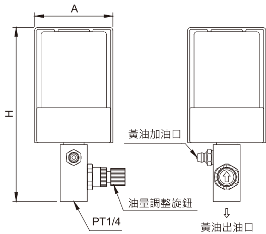
GP 外型圖
