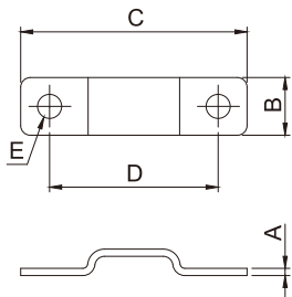
上座外型圖
