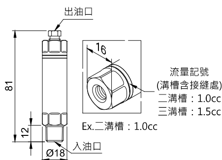
CCB-1 外型圖
