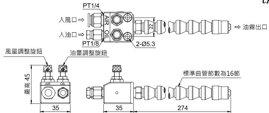
OT 噴槍外型圖
